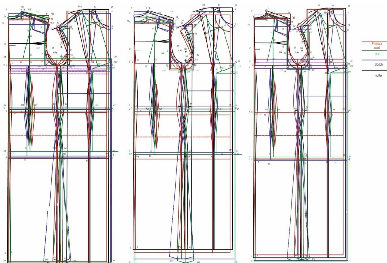
3-rasm. Fransuz, EMKO CƏB, Uinifred Aldrich va Müller & Sohn uslublari bo'yicha tayanch konstruksiyalarning ustma-ust tushishi va o'miz, ko'krak vabel chizig'ining konstanta sifatida mos kelishi
