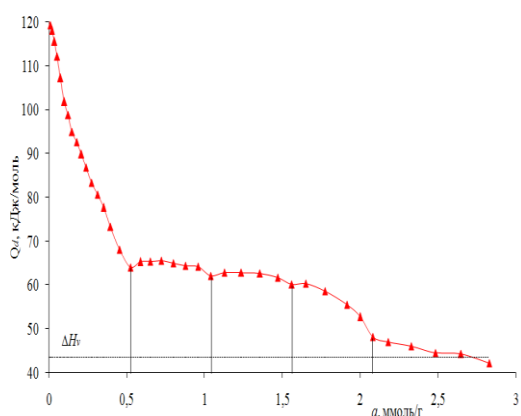
1-Расм. 303 К да гибрид диацетатцеллюлоза-кремнезем бионанокомпозицион материалга сувни адсорбциясининг дифференциал иссиқликлари: горизонтал штрихланган чизик - сувни конденсация иссиқлиги.
